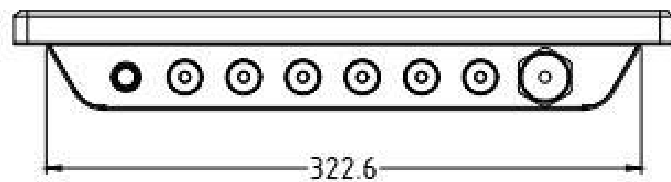
正视图
