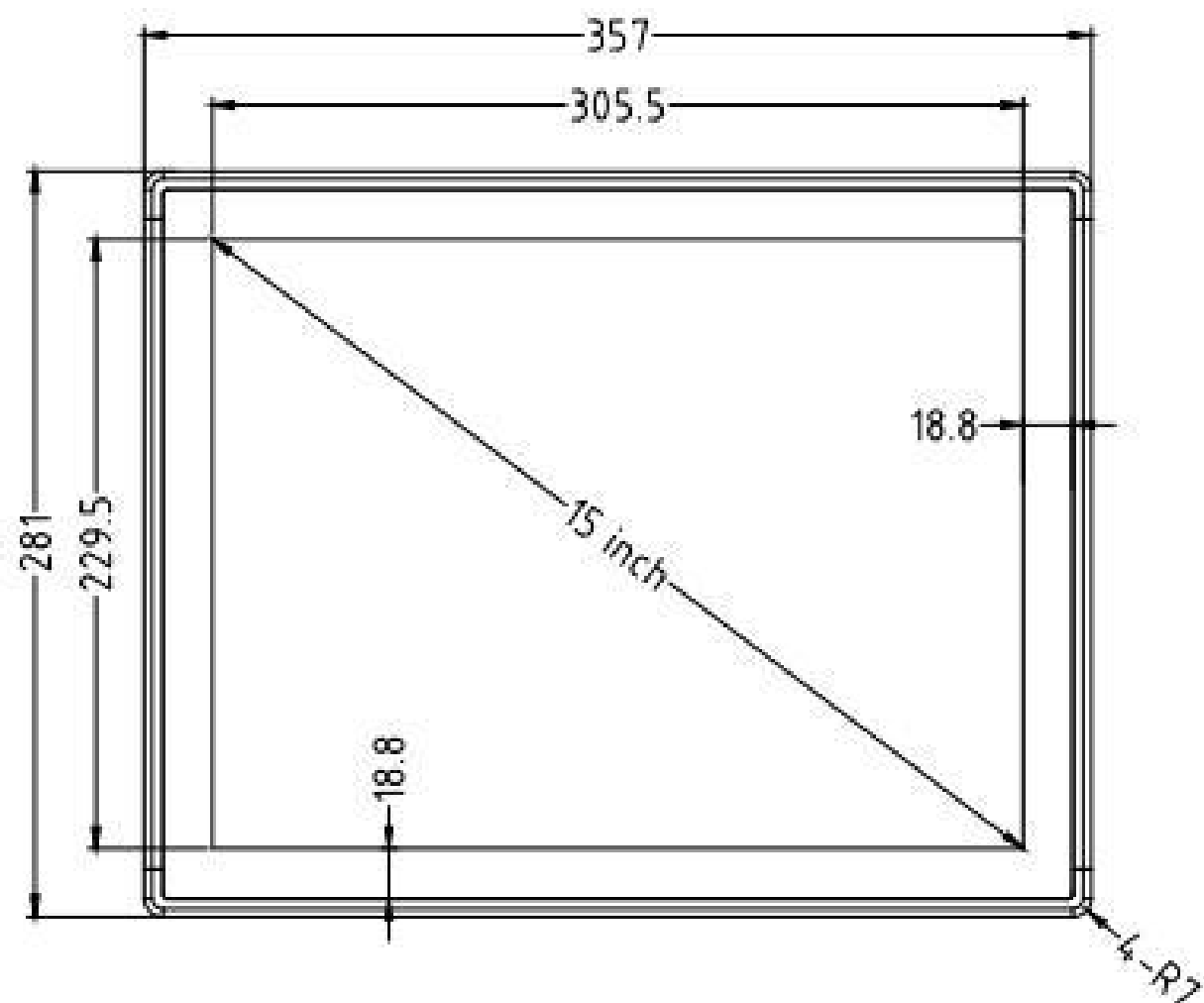
正视图
